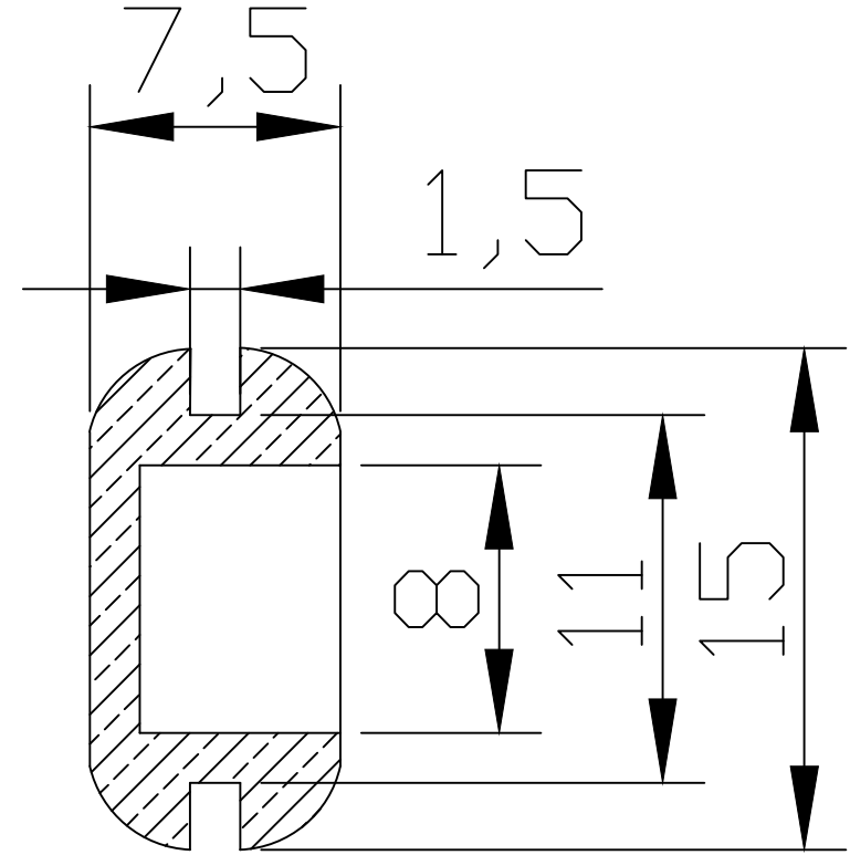
Sezione A-A
