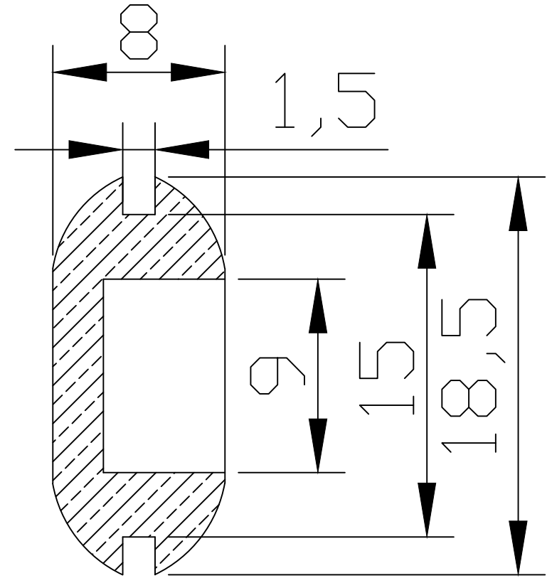
Sezione A-A
