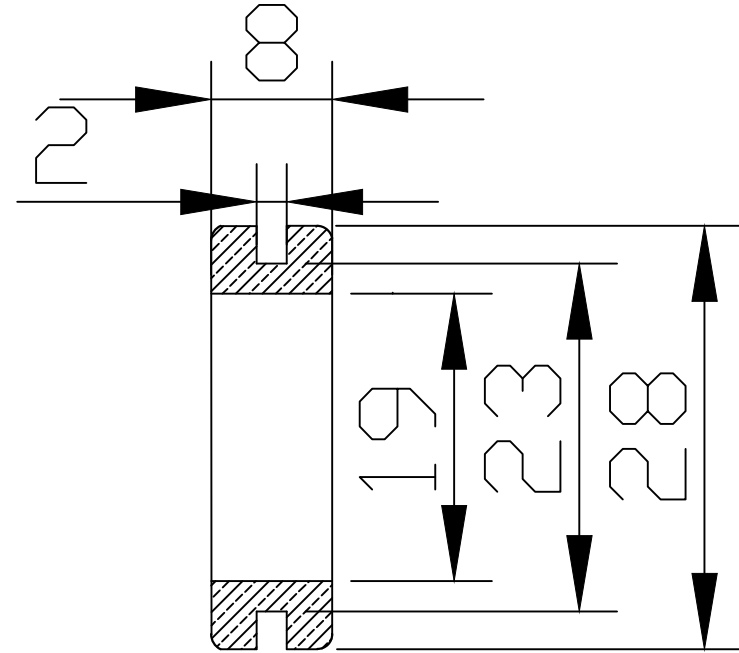
Sezione A-A
