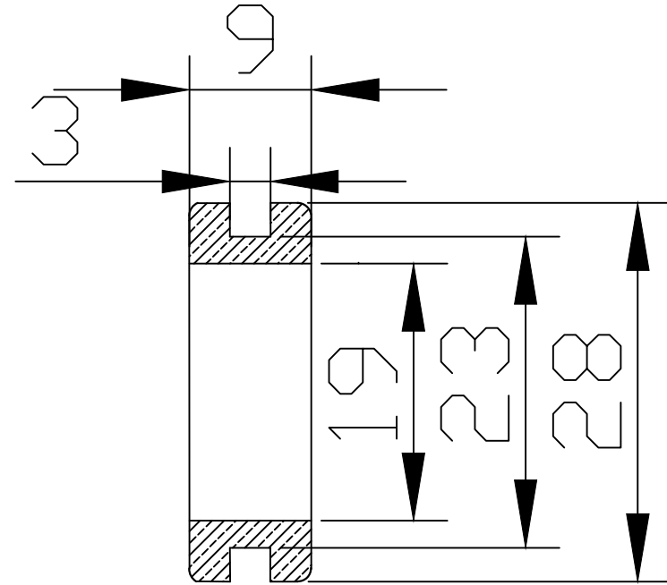
Sezione A-A
