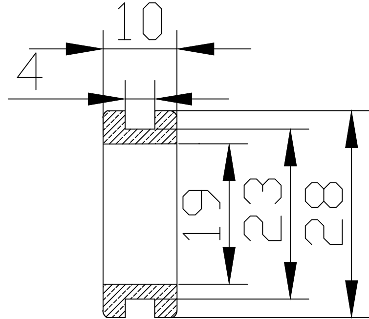
Sezione A-A
