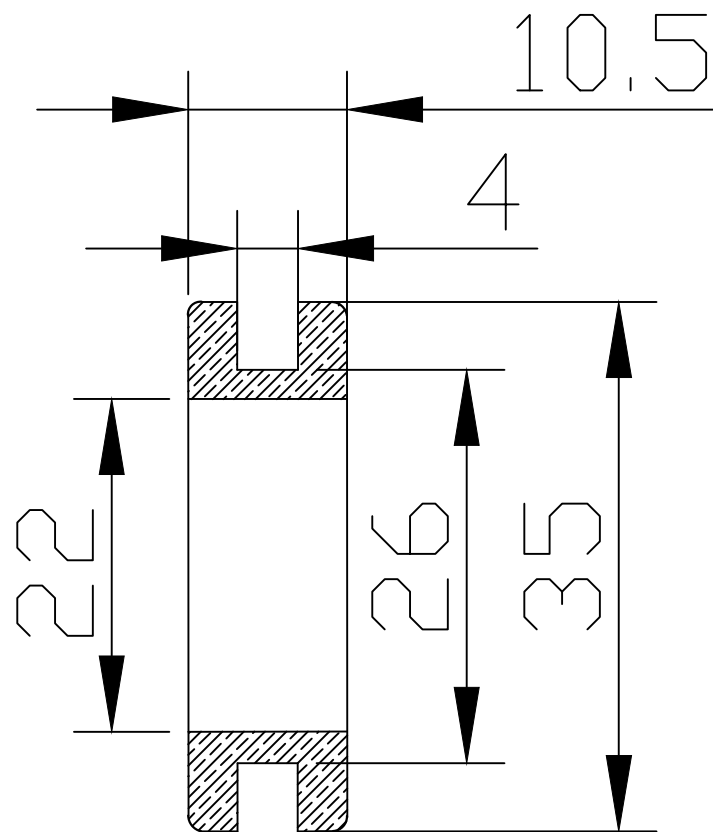
Sezione A-A
