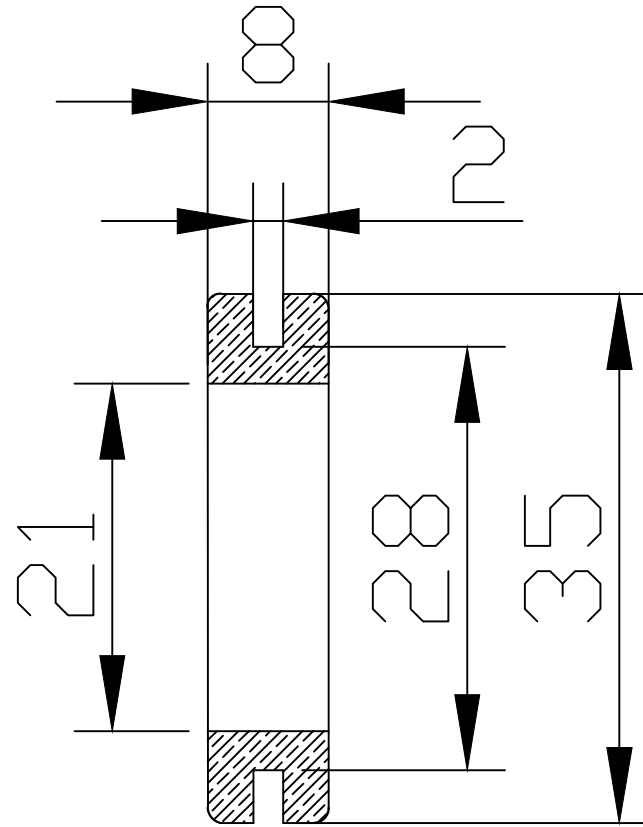
Sezione A-A
