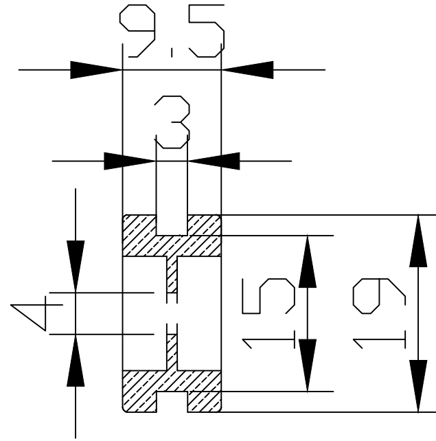
Sezione A-A
