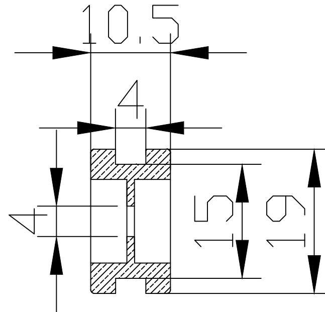
Sezione A-A
