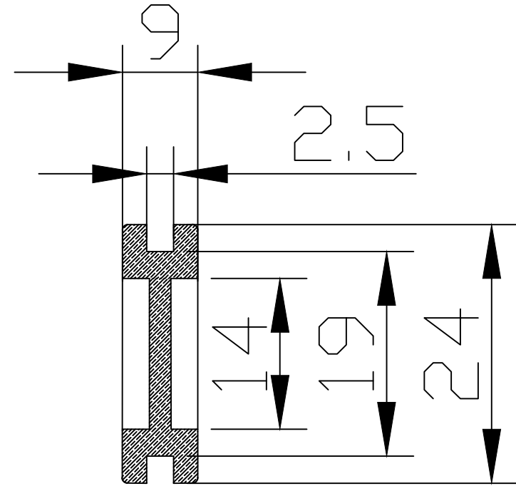
Sezione A-A
