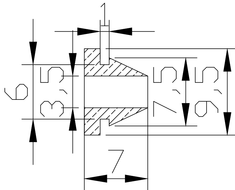
Sezione A-A
