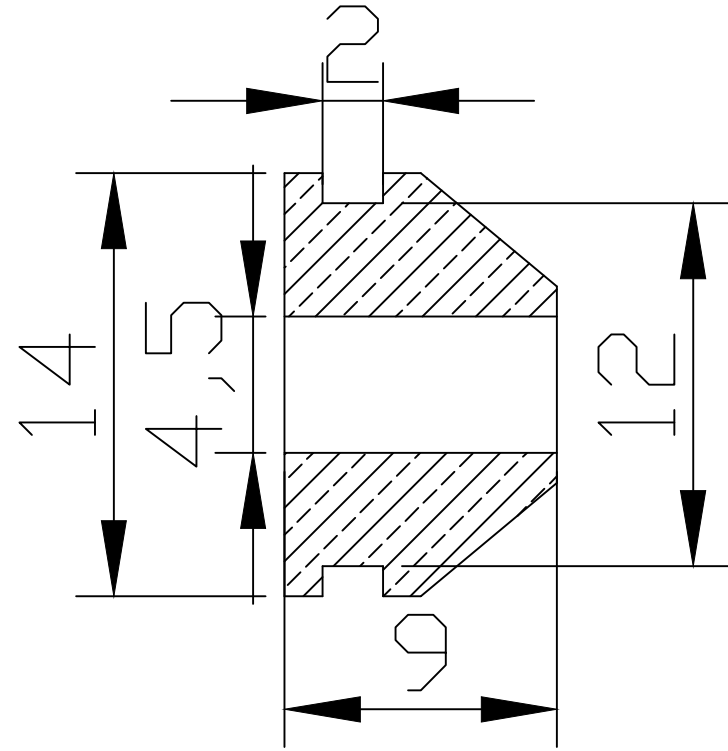
Sezione A-A
