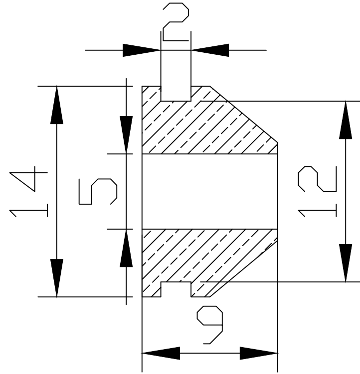
Sezione A-A
