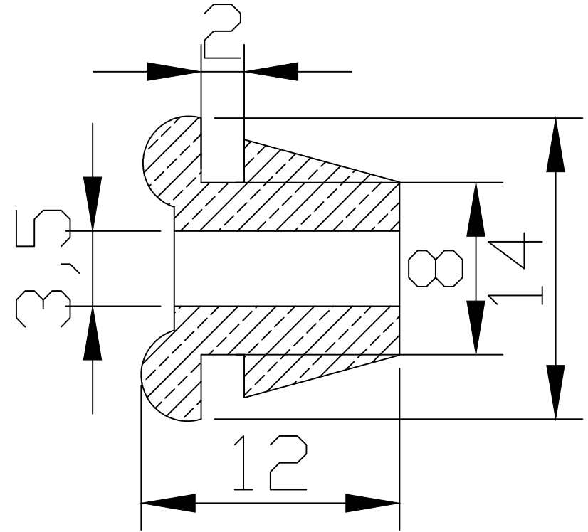
Sezione A-A
