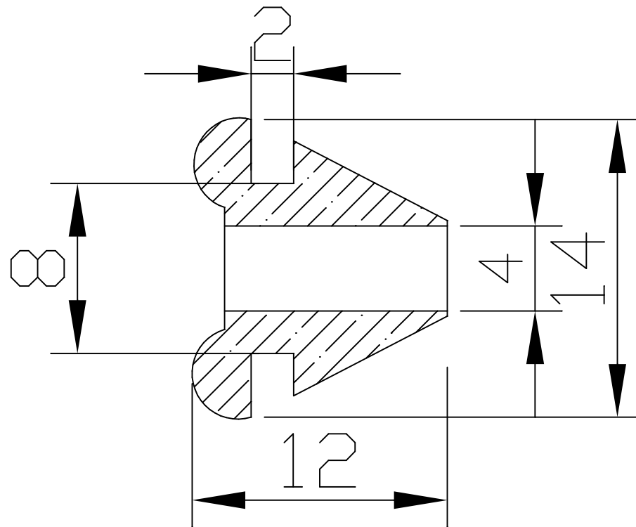
Sezione A-A
