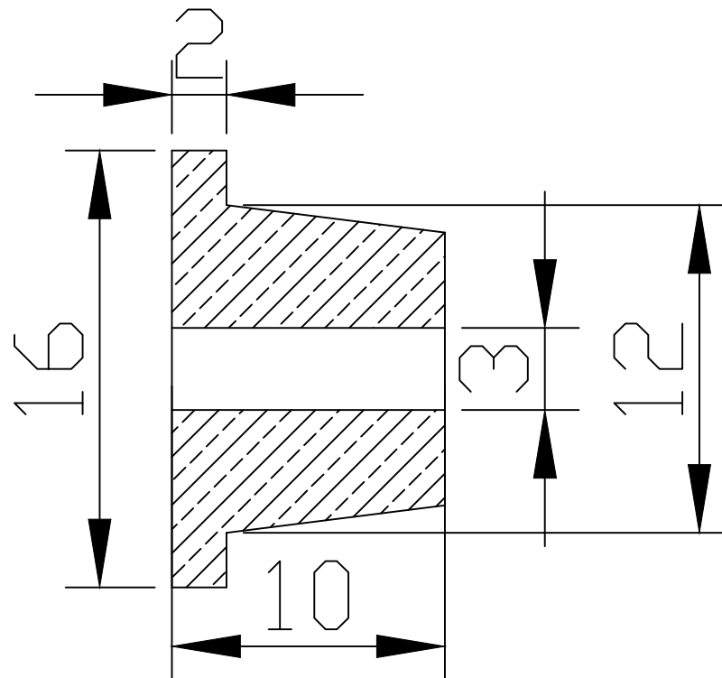
Sezione A-A
