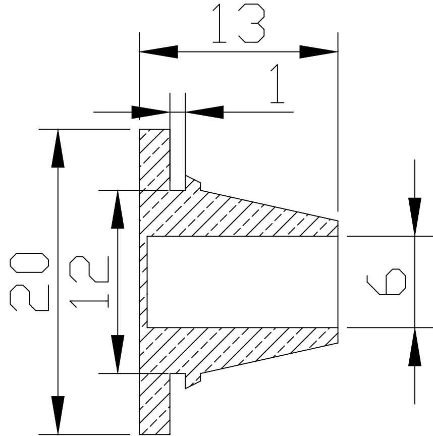
Sezione A-A
