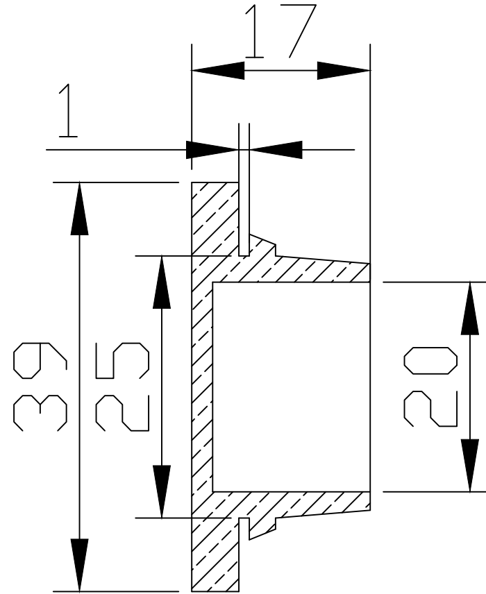
Sezione A-A
