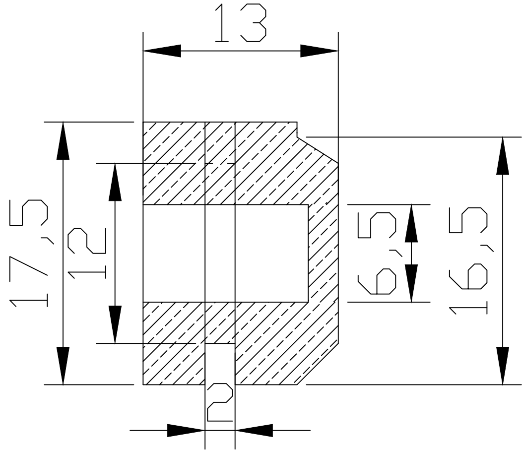
Sezione A-A
