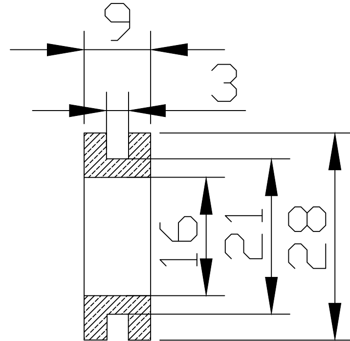
Sezione A-A
