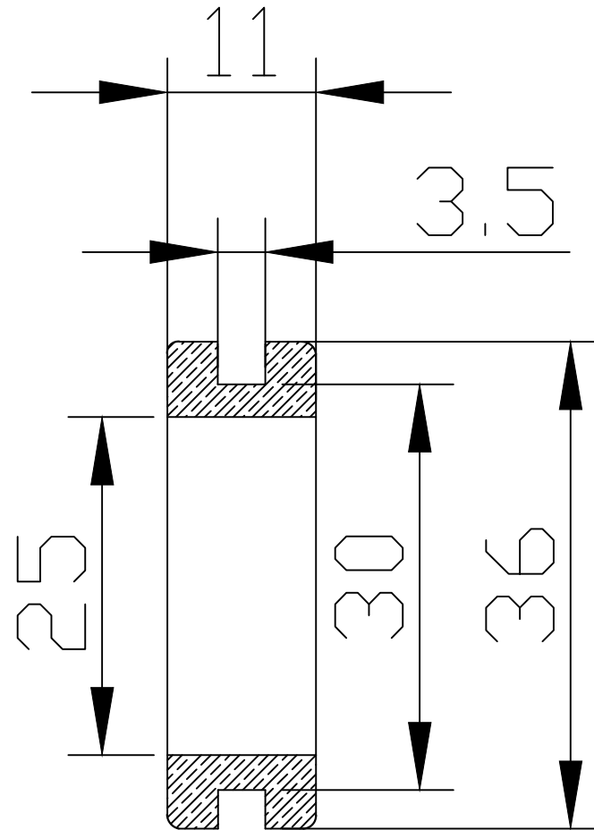
Sezione A-A
