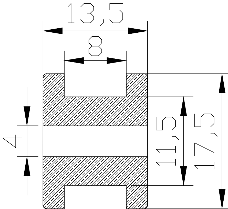
Sezione A-A
