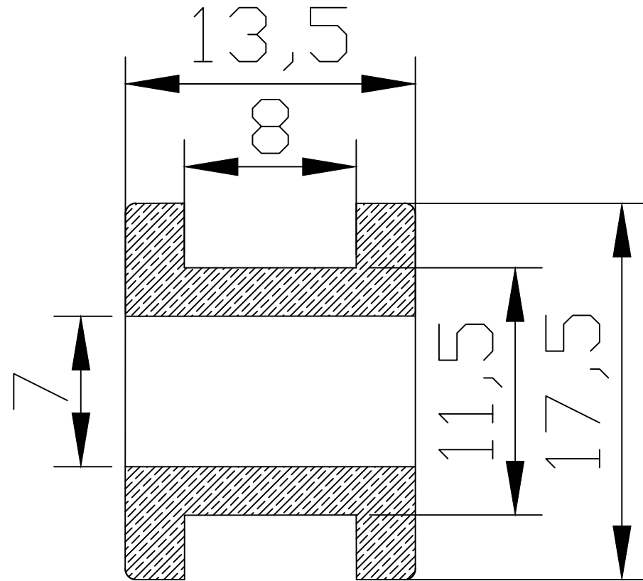
Sezione A-A
