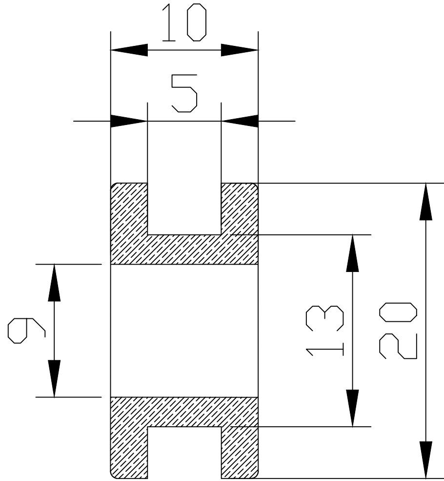
Sezione A-A
