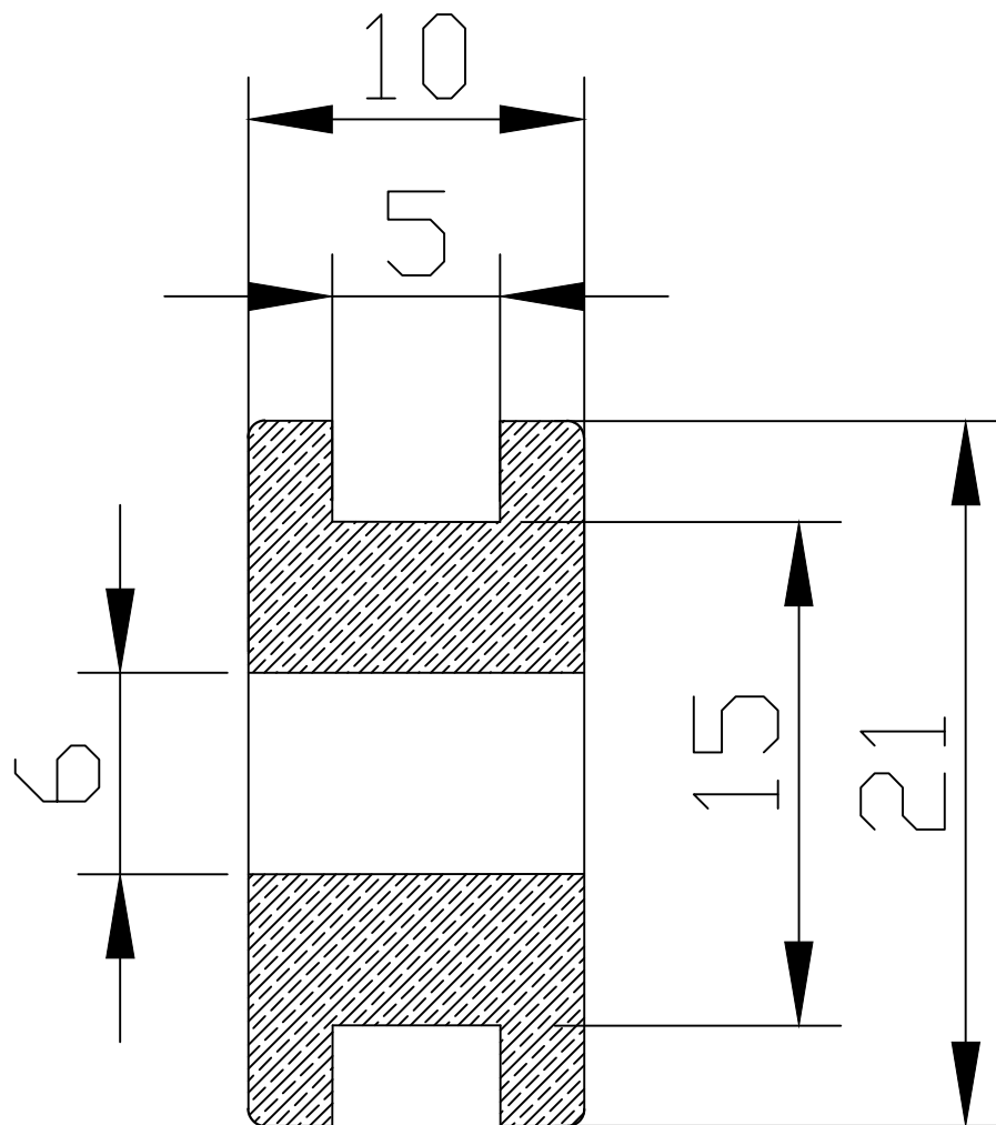
Sezione A-A
