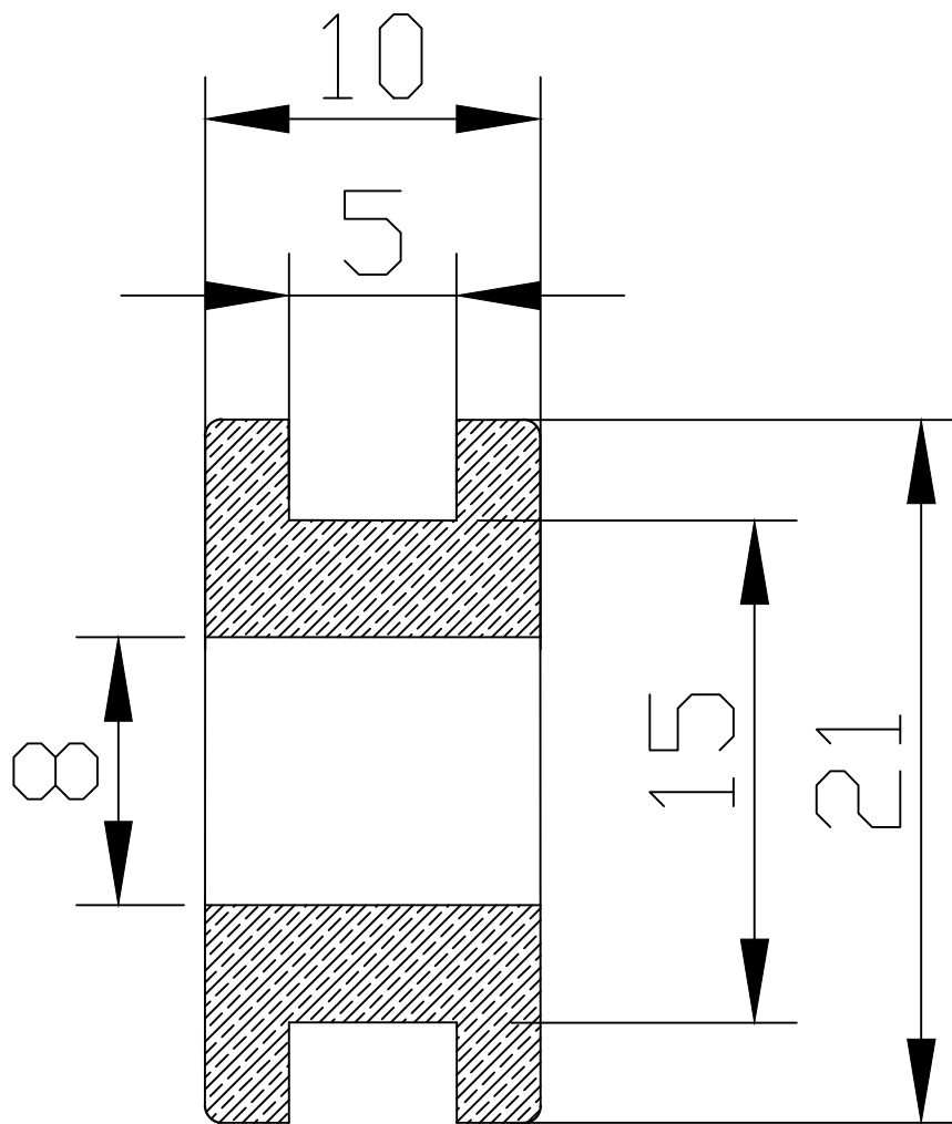
Sezione A-A
