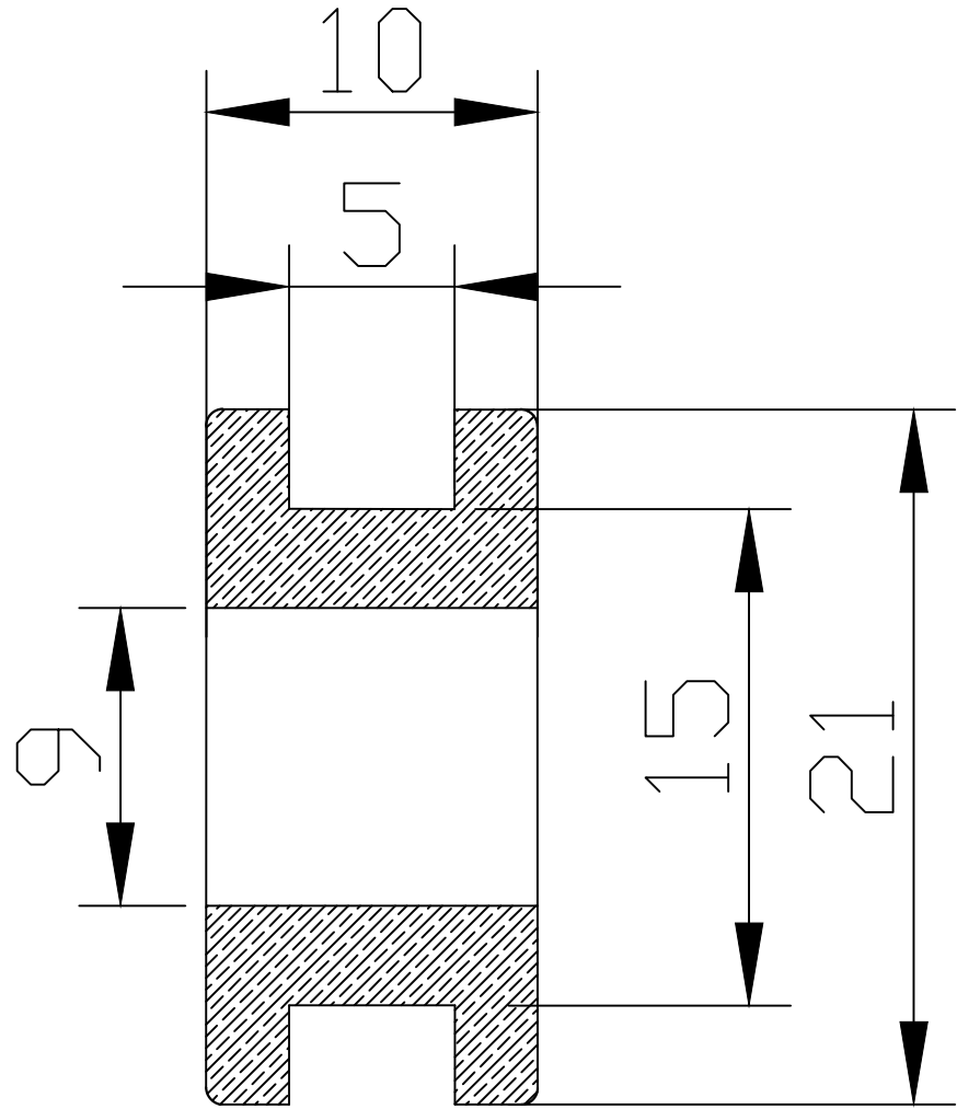
Sezione A-A
