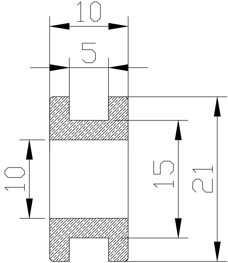
Sezione A-A
