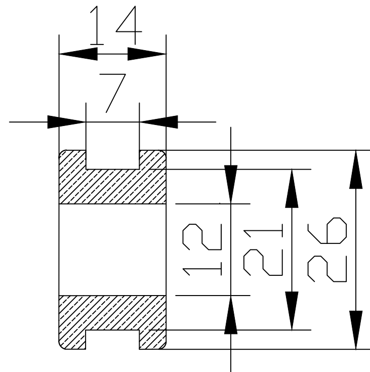
Sezione A-A
