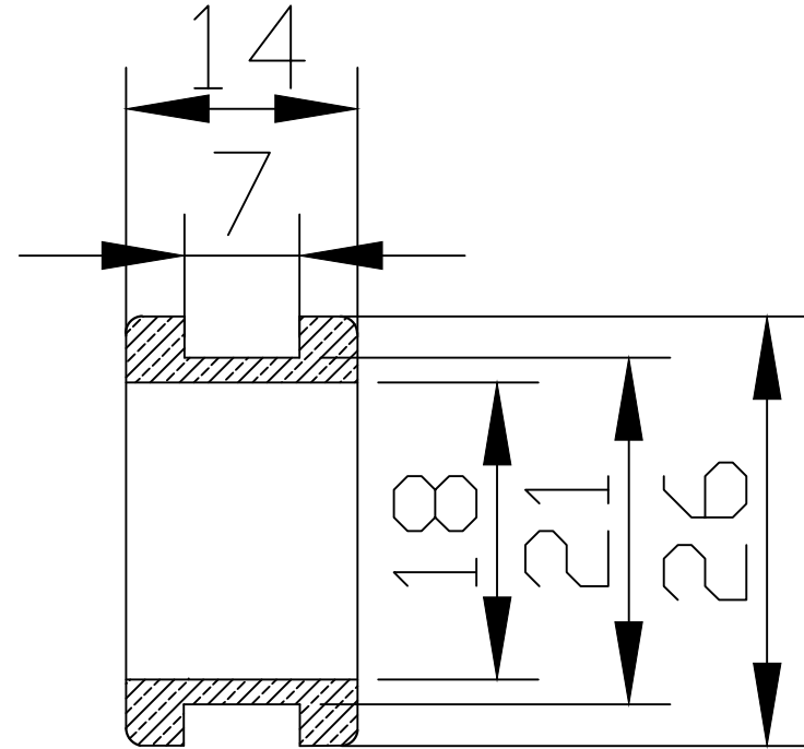
Sezione A-A
