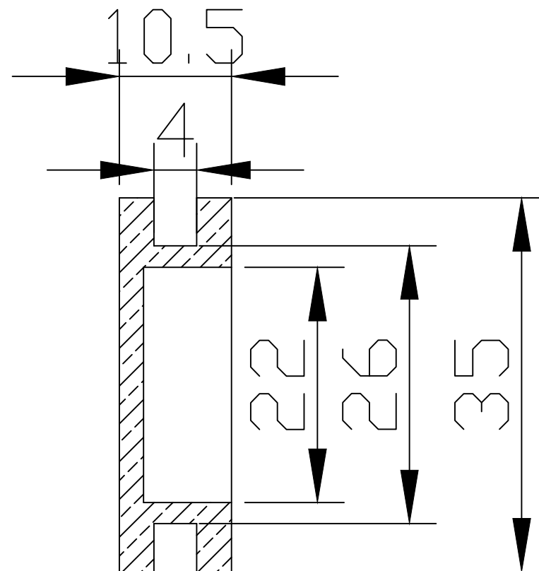
Sezione A-A
