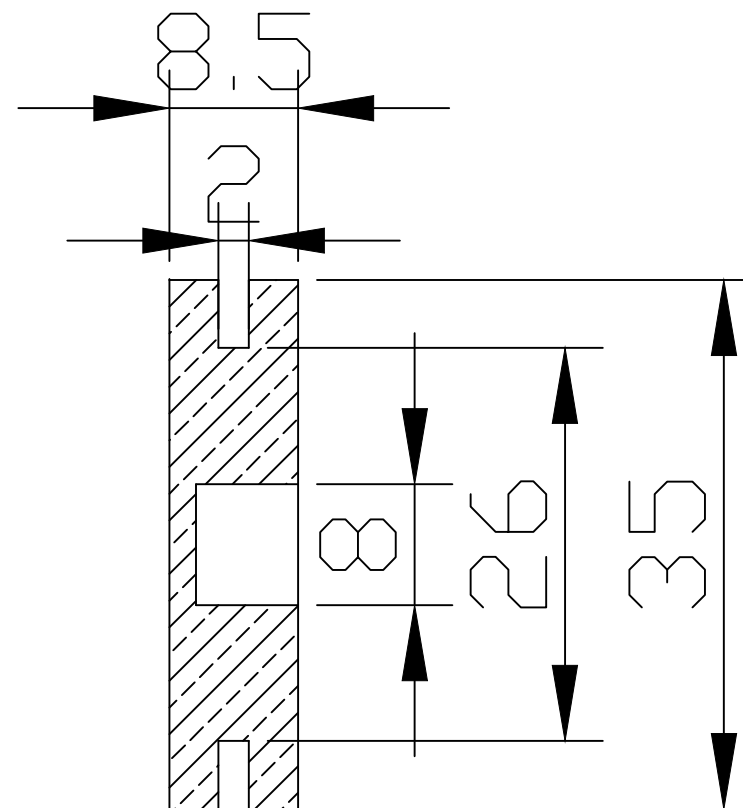
Sezione A-A
