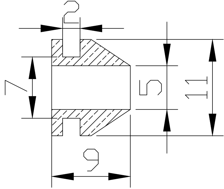
Sezione A-A
