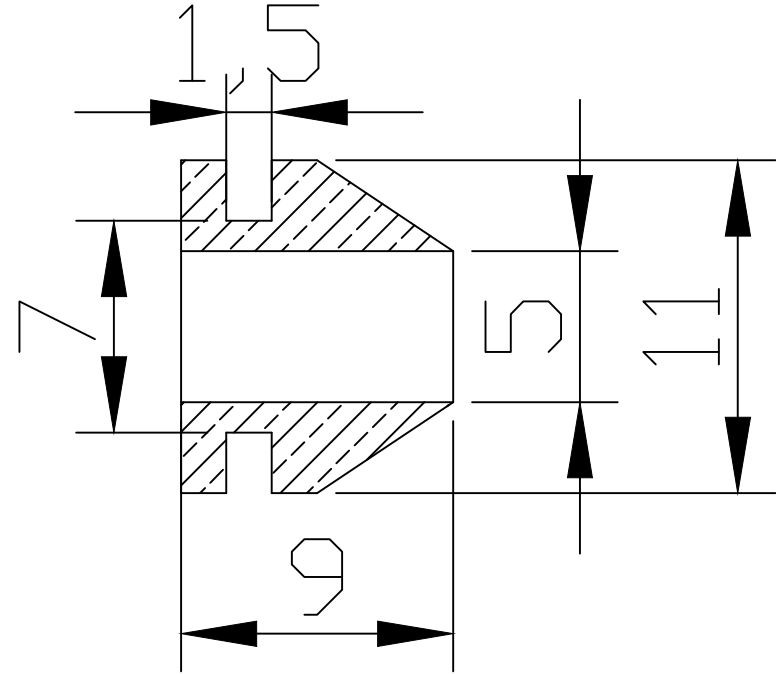
Sezione A-A
