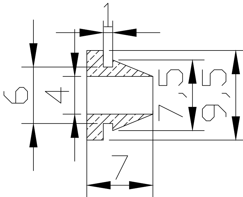
Sezione A-A
