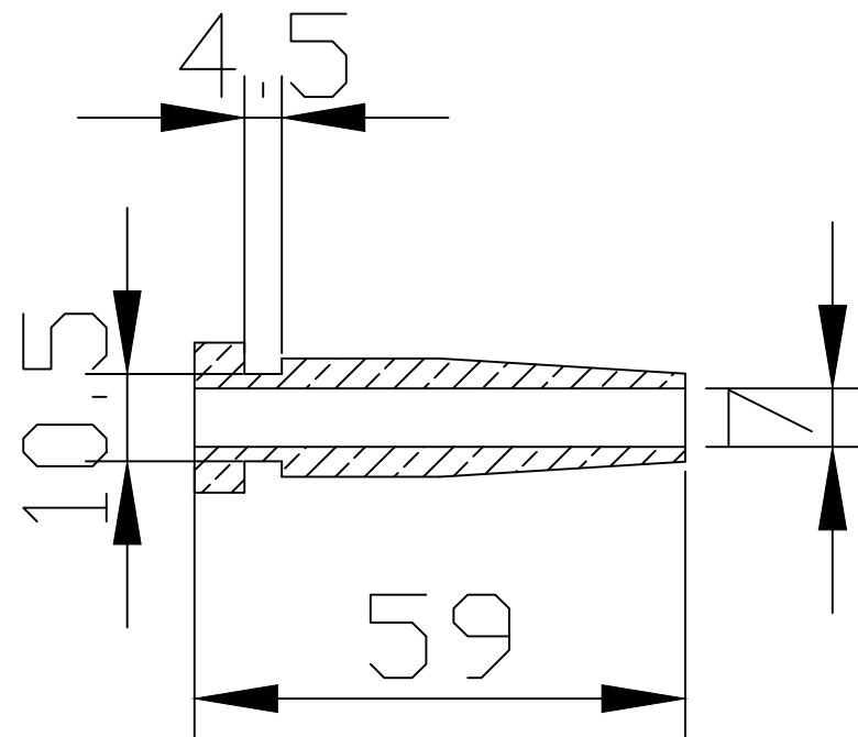
Sezione A-A
