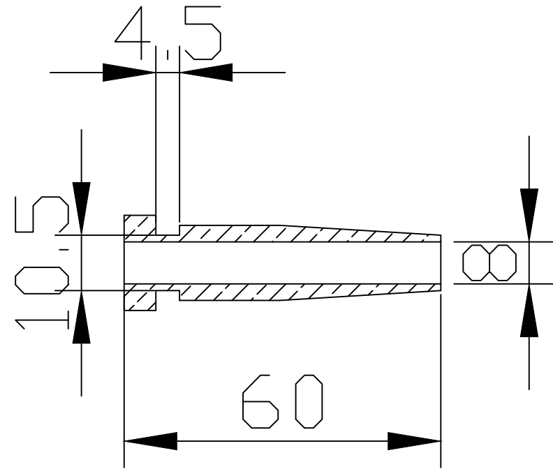
Sezione A-A
