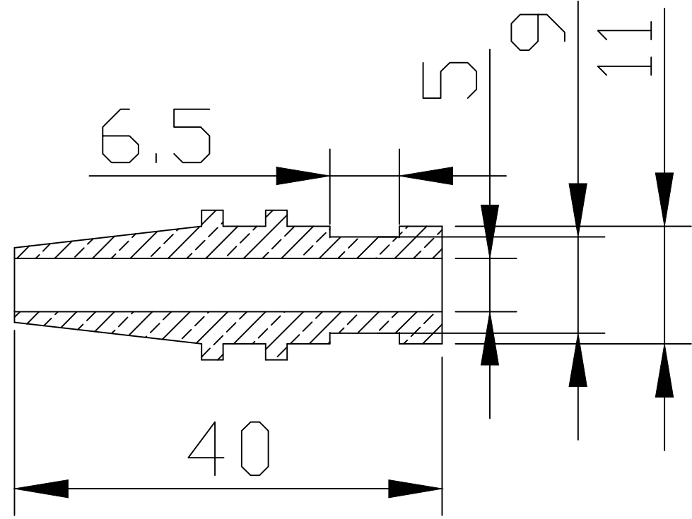
Sezione A-A
