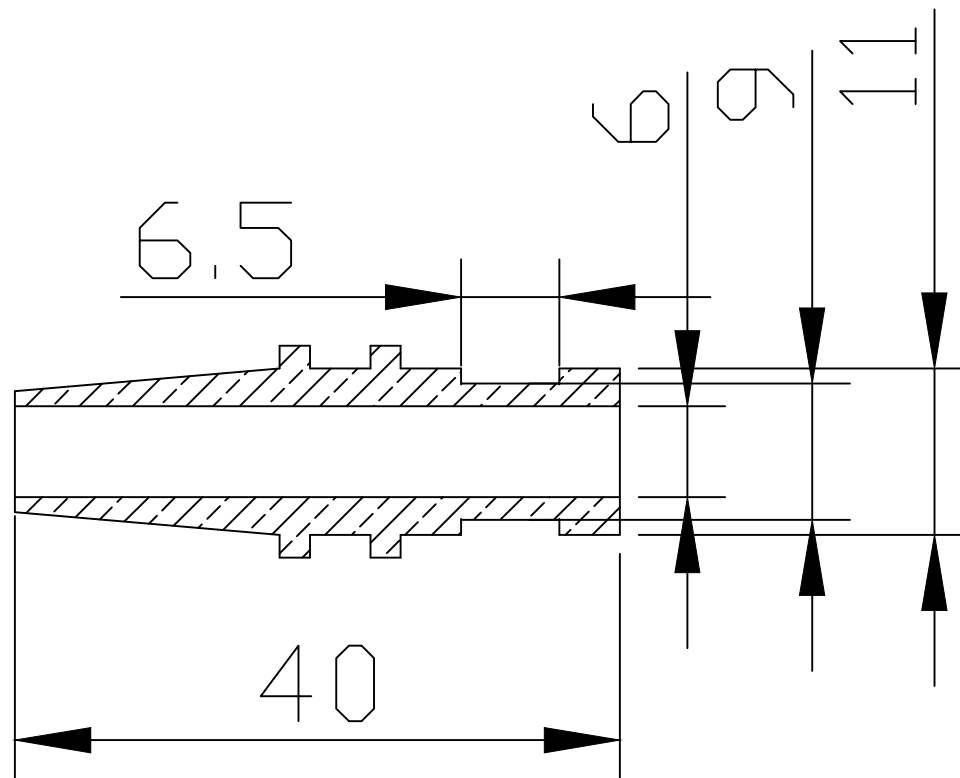
Sezione A-A
