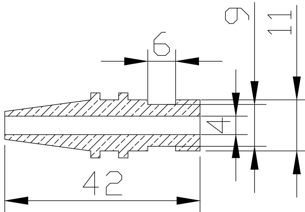
Sezione A-A
