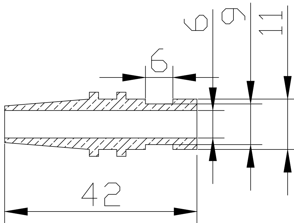
Sezione A-A
