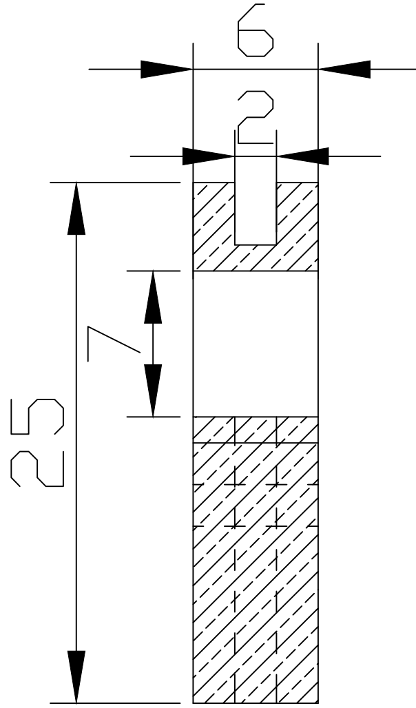
Sezione A-A
