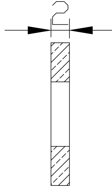
Sezione A-A
