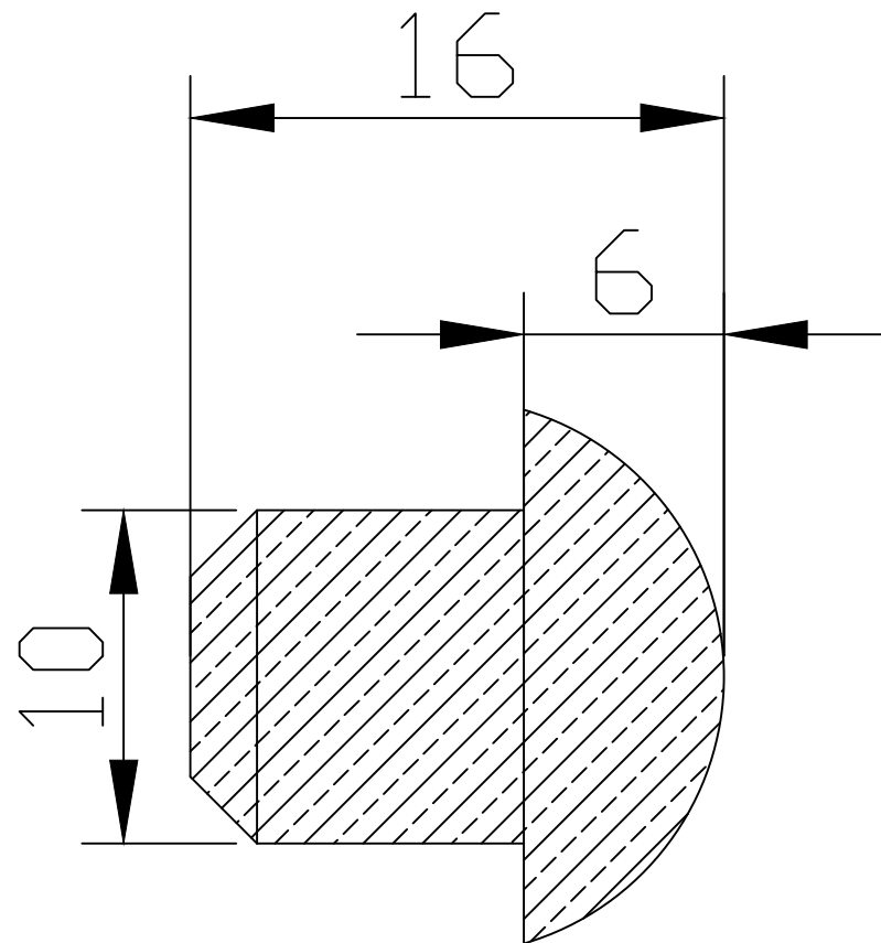
Sezione A-A
