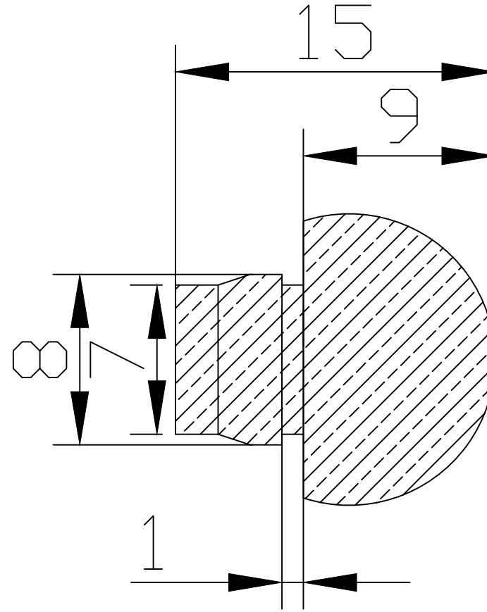
Sezione A-A
