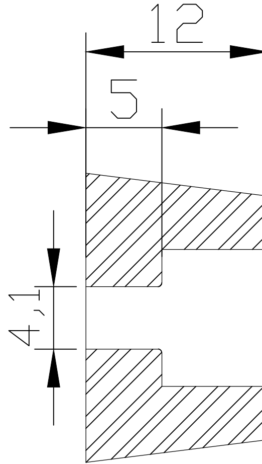
Sezione A-A
