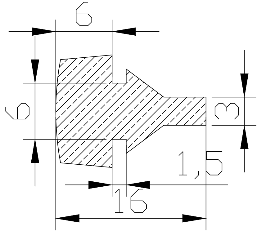
Sezione A-A
