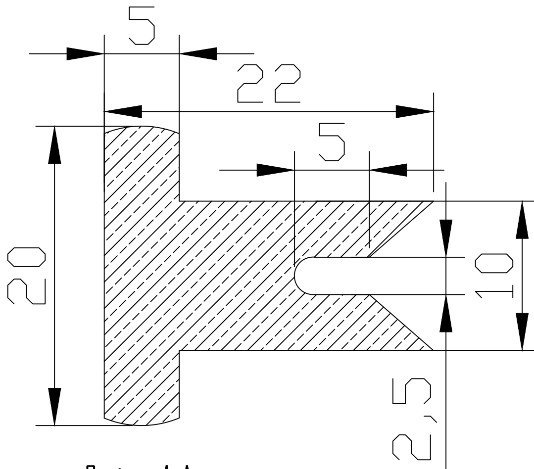
Sezione A-A
