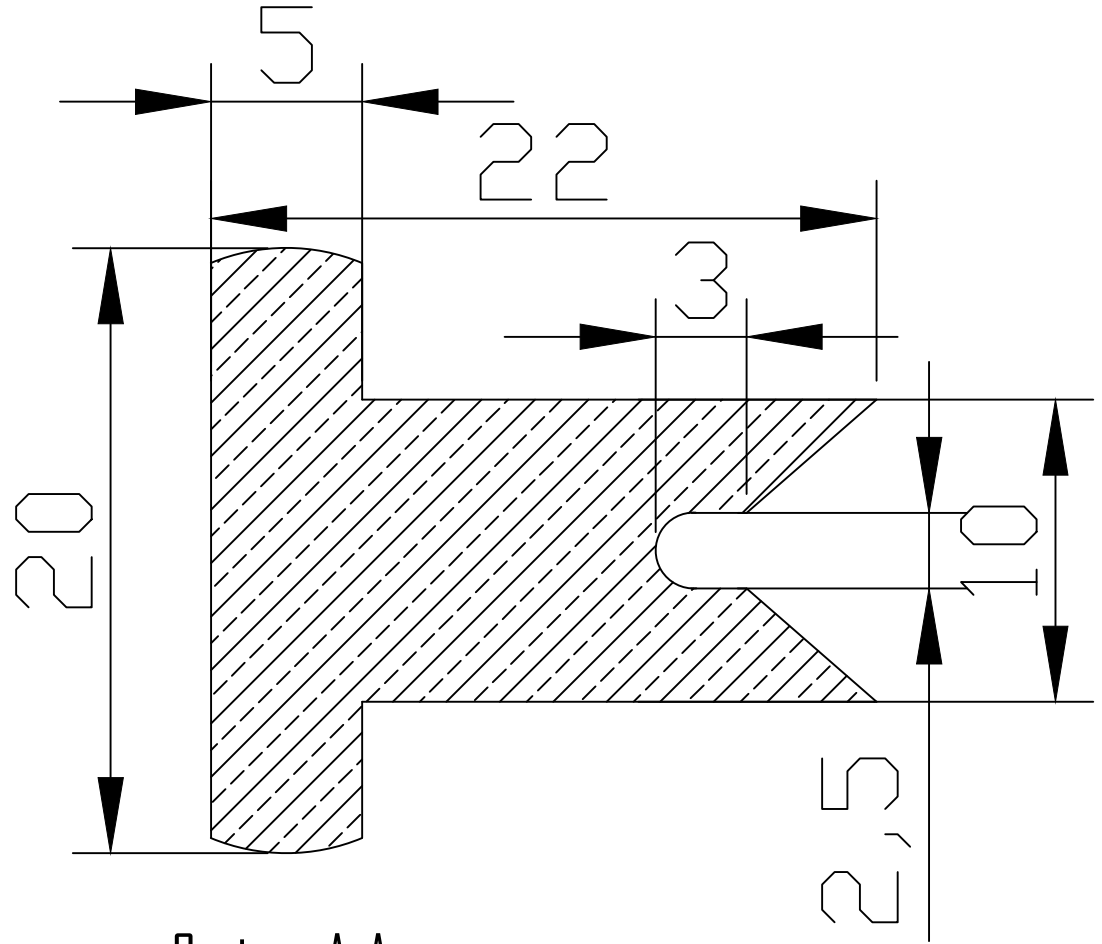
Sezione A-A
