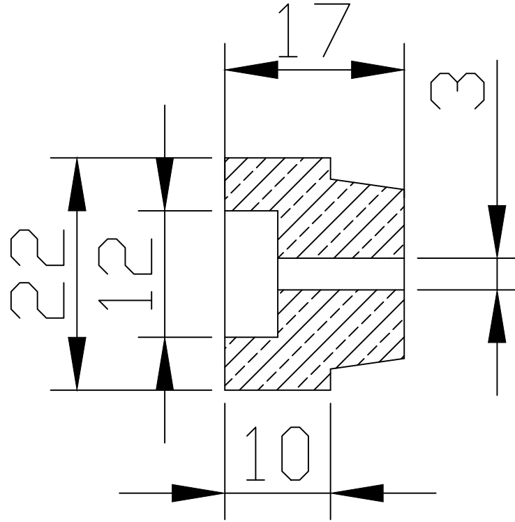
Sezione A-A
