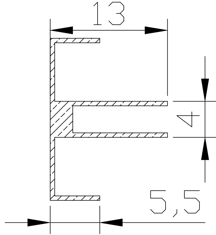
Sezione A-A
